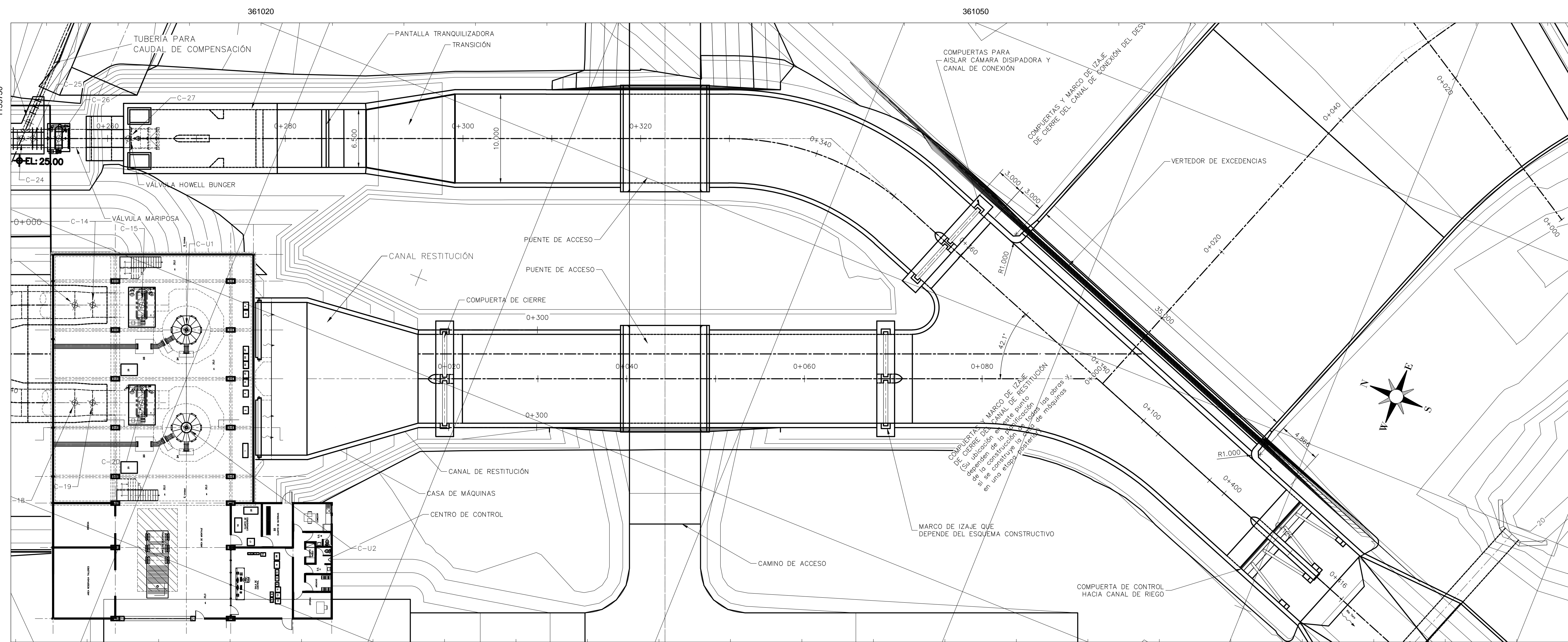
VISTA EN PLANTA DEL CANAL DE CONEXIÓN ENTRE LA CÁMARA DISIPADORA, ÁREA DE CONTROL Y CANAL DE RIEGO
